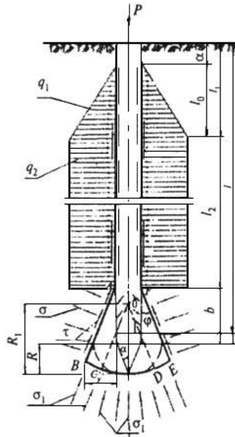
Рисунок Е.1 - Расчетная схема
