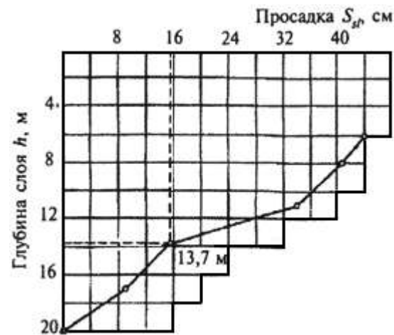
Рисунок Е.2 - График зависимости S_{sl} = f(h)
